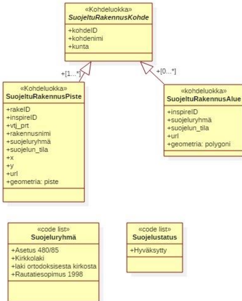
Kuva 2. Suojeltujen rakennusten aineiston (rakennusperintörekisteri) rakenne ja tietokentät
